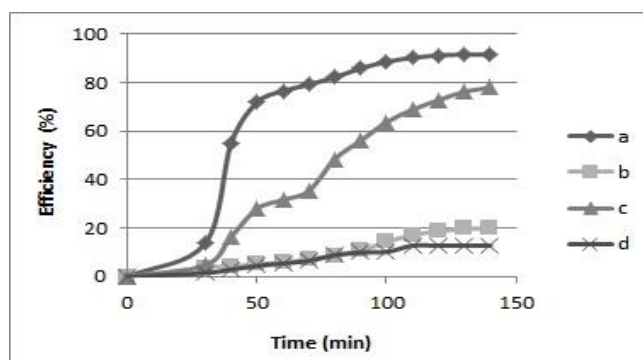
شکل ۷. راندمان حذف کاتالیستی با 3/9 \text{ w/m}^2 شدت تابش فرابنفش (a) \text{TiO}_2/\text{Zeolite} با غلظت 10 \text{ mg/L} ؛ (b) \text{TiO}_2 با غلظت 10 \text{ mg/L} ؛ (c) \text{TiO}_2/\text{Zeolite} با غلظت 50 \text{ mg/L} ؛ (d) \text{TiO}_2 با غلظت 50 \text{ mg/L}
