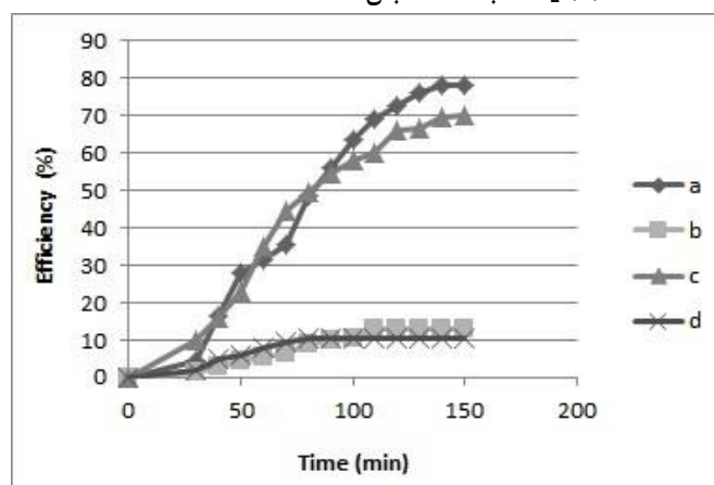
شکل ۶. راندمان حذف فتوکاتالیستی با غلظت 50 \text{ mg/L} (a) \text{TiO}_2/\text{Zeolite} با شدت تابش 3/9 \text{ w/m}^2 ؛ (b) \text{TiO}_2 با شدت تابش 3/9 \text{ w/m}^2 ؛ (c) \text{TiO}_2/\text{Zeolite} با شدت تابش 2/4 \text{ w/m}^2 ؛ (d) \text{TiO}_2 با شدت تابش 2/4 \text{ w/m}^2
