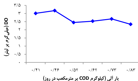
شکل ۵. روند تغییرات غلظت DO (Dissolved oxygen)
