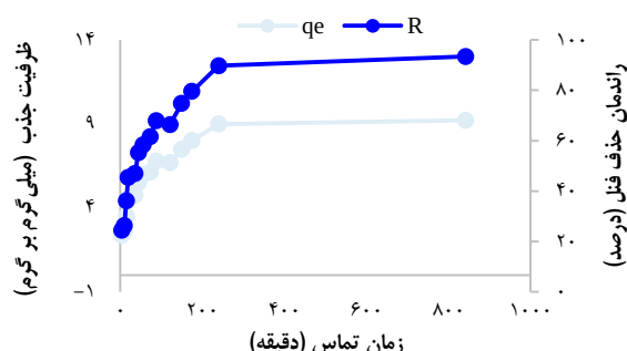
شکل ۲. تأثیر زمان تماس بر راندمان حذف فنل (غلظت اولیه فنل = ۱۰ میلی‌گرم بر لیتر، دوز کربن فعال = ۱ گرم بر لیتر و pH = ۷)
