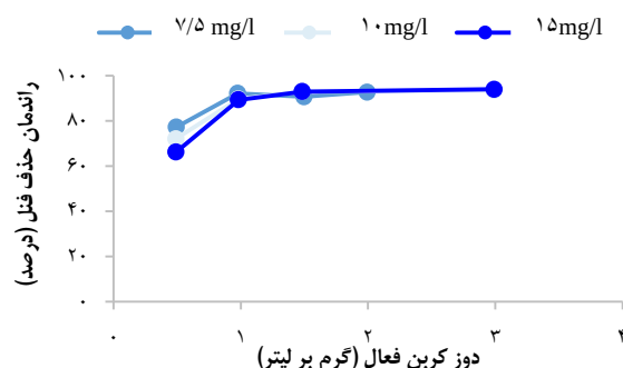
شکل ۳. کارایی حذف فنل با استفاده از کربن فعال به عنوان تابعی از دوز کربن فعال و غلظت اولیه فنل ( pH = 7 و زمان تماس = ۸۴۰ دقیقه)
