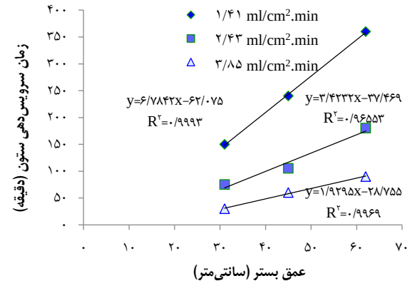
شکل ۳. زمان کارکرد ستون‌های جاذب GAC (Granular activated carbon) بر حسب تغییرات عمق ستون
